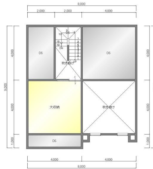
M2階 平面図
