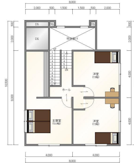
2階 平面図
