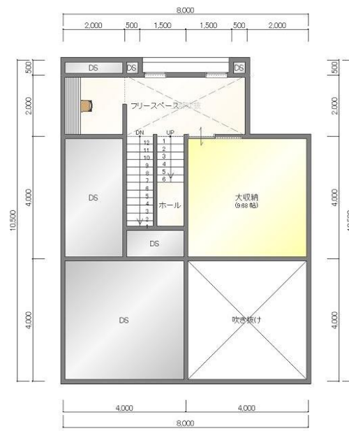
M2階 平面図
